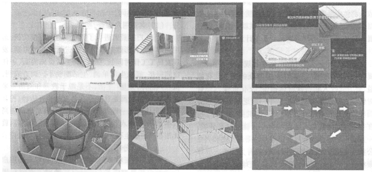
图1 可周转、易回收、预制型农民工用住宅产品设计
