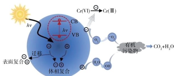
图 1 g\text{-C}_3\text{N}_4 的光降解污染物、金属 Cr 的机理
