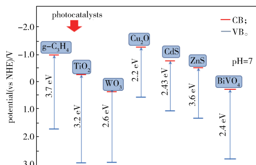
图 3 常见的半导体光催化剂的能带结构图
